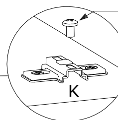
parafuso fixador tornillo fijador fixer bolt DETALHE 5 DETALLE 5 DETAIL 5
